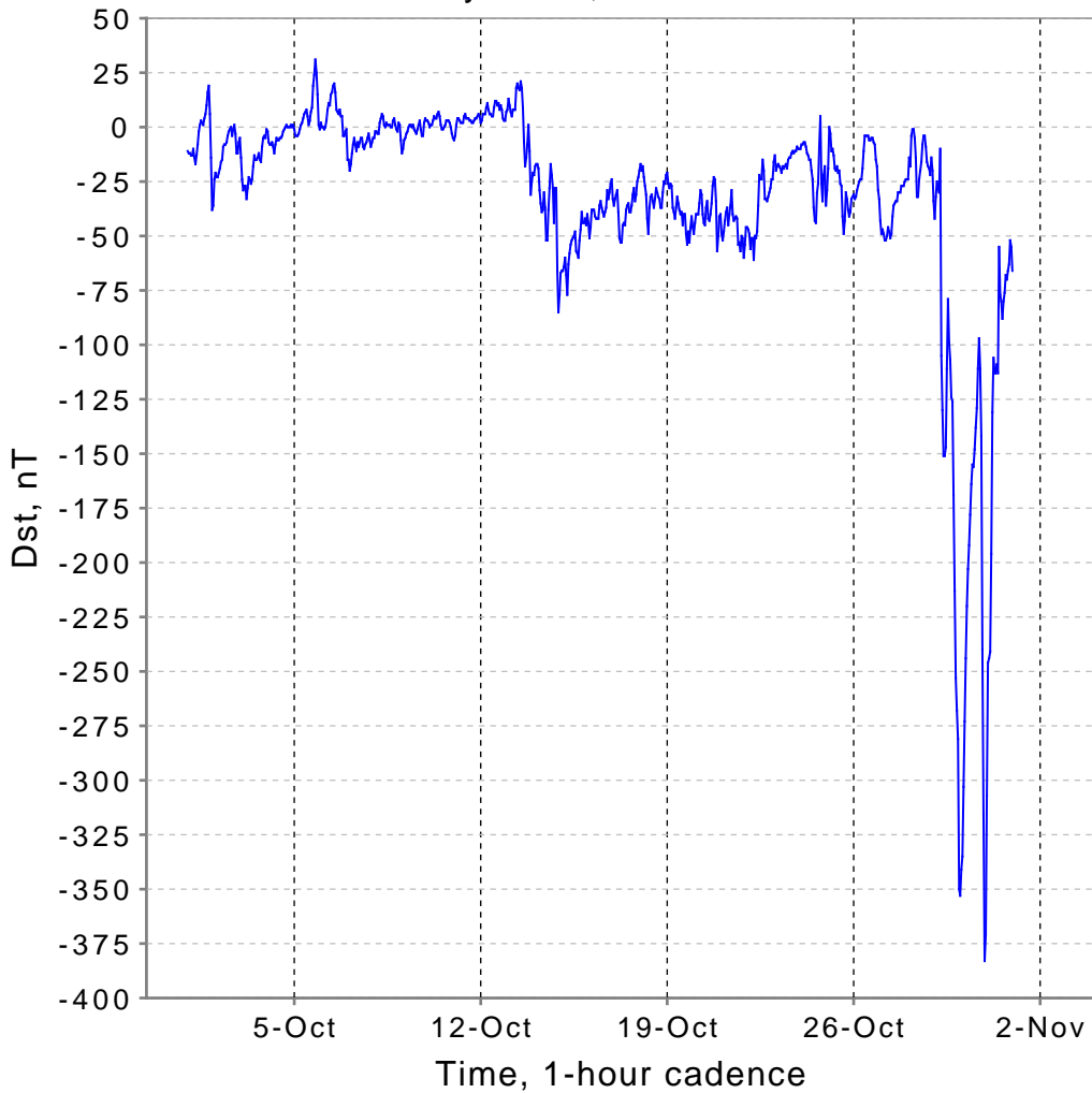
Kyoto Dst, nT
